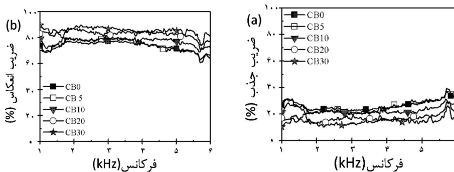
شکل ۹ - اثر دوده بر خواص صوتی اسفنج‌های NR (a) ضریب جذب و (b) ضریب انعکاسی امواج صدا
