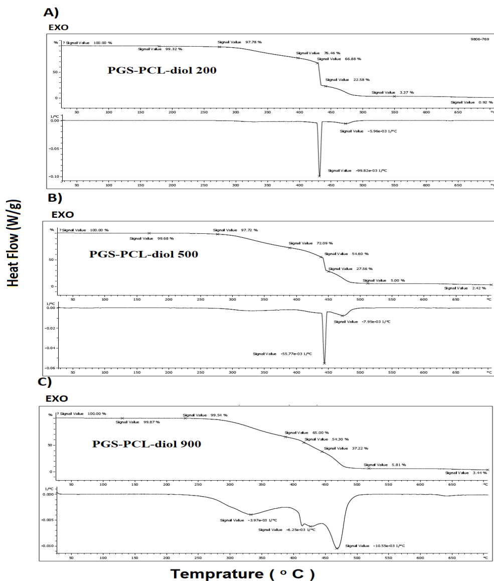
شکل ۴ تصویر تحلیل DSC نمونه داربست‌های (A PGS-PCL-diol 200، B PGS-PCL-diol 500، C PGS-PCL-diol 900) Figure 4 DSC analysis image of PGS-PCL-diol 200 scaffolds (A, B, PGS-PCL-diol 500, C) PGS-PCL-diol 900
