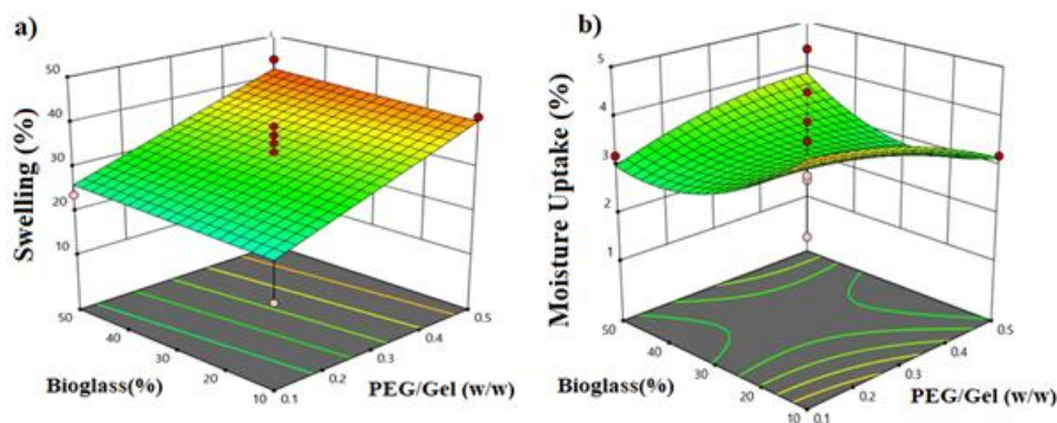
شکل ۳ نمودار سطح پاسخ الف) درصد جذب رطوبت ب) درصد تورم بر حسب نسبت وزن PEG/Gel و درصد وزنی BG
