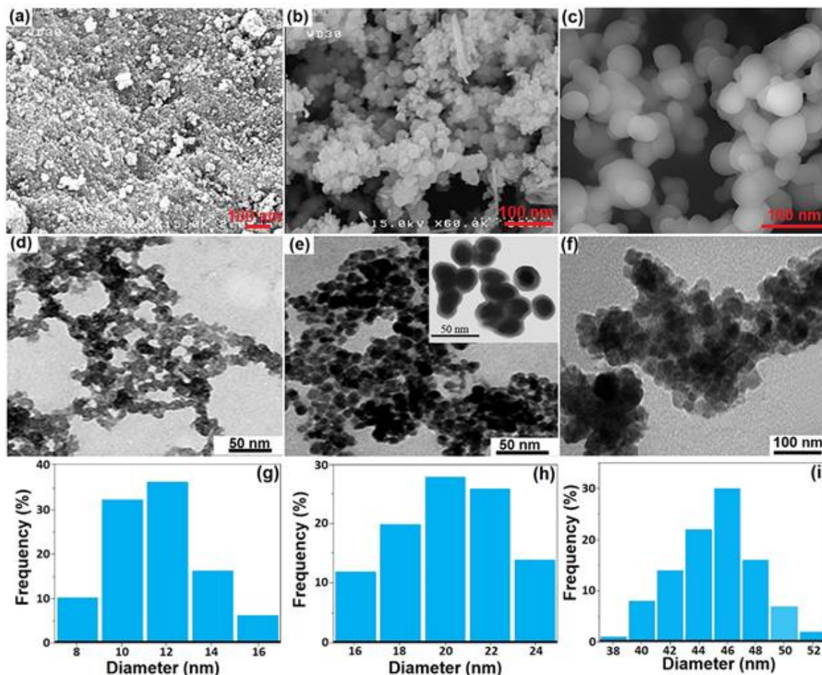
شکل ۴ تصاویر میکروسکوپی الکترونی پویشی نانوذرات (a) Fe 3 O 4 , (b) Fe 3 O 4 @SiO 2 و (c) Fe 3 O 4 @SiO 2 -TCT-PVA، تصاویر میکروسکوپی الکترونی عبوری نانوذرات (d) Fe 3 O 4 , (e) Fe 3 O 4 @SiO 2 و (f) Fe 3 O 4 @SiO 2 -TCT-PVA. توزیع اندازه ذرات (g) Fe 3 O 4 و (h) Fe 3 O 4 @SiO 2 و (i) Fe 3 O 4 @SiO 2 -TCT-PVA
