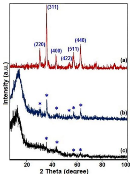
شکل ۳ پراش پرتوی ایکس نانوذرات سنتزی (a) \text{Fe}_3\text{O}_4 ، (b) \text{Fe}_3\text{O}_4/\text{SiO}_2 و \text{Fe}_3\text{O}_4/\text{SiO}_2 -TCT-PVA (c)
