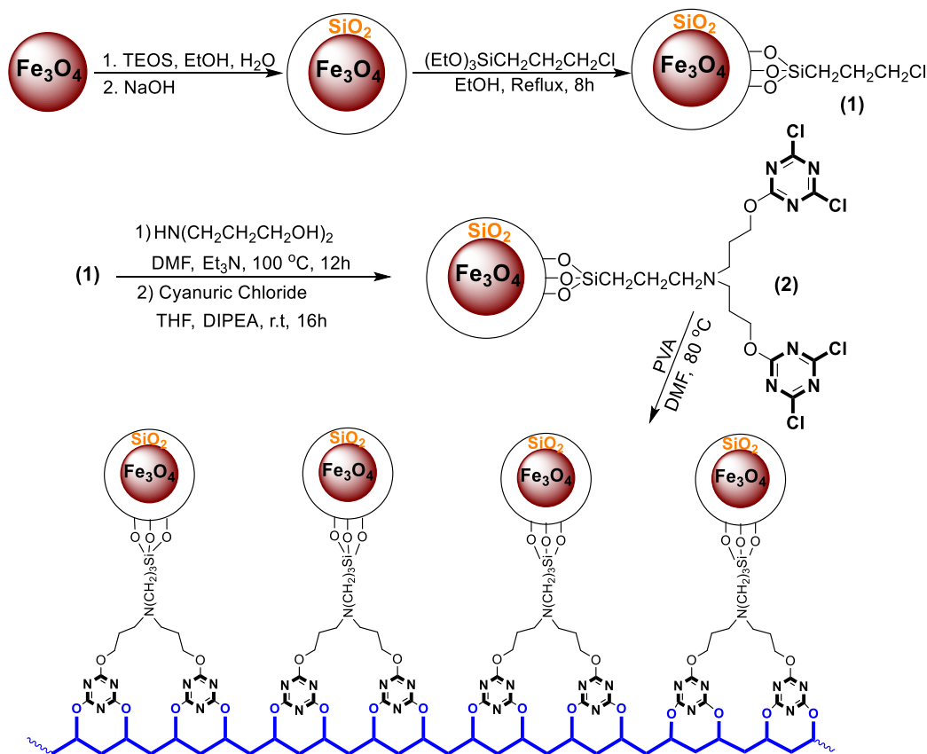
شکل ۱ طرح‌واره سنتز مرحله به مرحله عامل‌دار شدن نانوذرات \text{Fe}_3\text{O}_4@/\text{SiO}_2 با پلی‌وینیل الکل Figure 1 The schematic of step-to-step functionalization of \text{Fe}_3\text{O}_4@/\text{SiO}_2 with polyvinyl alcohol
