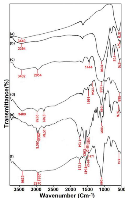
شکل ۲ طیف‌سنجی فروسرخ تبدیل فوری نانوذرات (a) \text{Fe}_3\text{O}_4 ، (b) \text{Fe}_3\text{O}_4/\text{SiO}_2 ، (c) \text{Fe}_3\text{O}_4/\text{SiO}_2 -Cl، (d) \text{Fe}_3\text{O}_4/\text{SiO}_2 -N(OH) _2 ، (e) \text{Fe}_3\text{O}_4/\text{SiO}_2 -TCT، و (f) \text{Fe}_3\text{O}_4/\text{SiO}_2 -TCT-PVA
