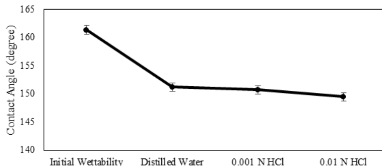
شکل ۷ اثر آب مقطر و محلول‌های اسیدی بر زاویه تماس Figure 7. Effect of distilled water and acidic solutions on contact angle
