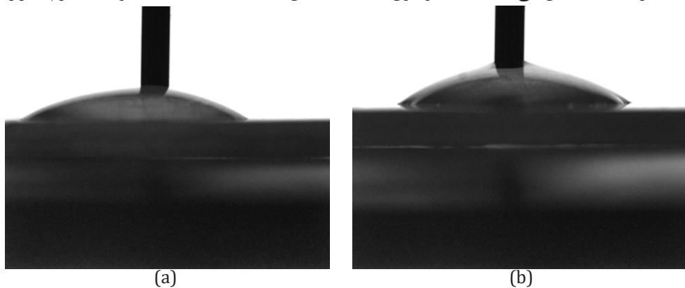
شکل ۶. تصاویر آزمون سطح تماس الف- قبل و ب- بعد از تابش پلازما Fig 6. CA images of PP (a) before and (b) after plasma irradiation.
