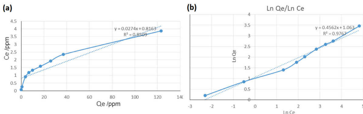
شکل ۶ (a) همدمای جذب لانگمویر و (b) همدمای جذب فرندلیچ یون‌های \text{Cu(II)} بر روی جاذب
