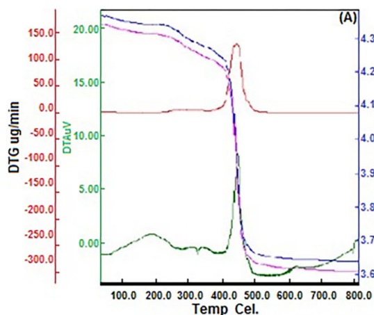
شکل ۳ (A) الگوی آزمون توزین حرارتی \text{MnFe}_2\text{O}_4@\text{SiO}_2@\text{PMIDA} . (B) تصویر VSM نانوذرات (a) \text{MnFe}_2\text{O}_4 و (b) \text{MnFe}_2\text{O}_4@\text{SiO}_2@\text{PMIDA}
