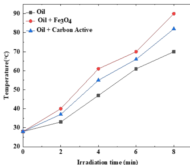
شکل ۷ تغییرات دما در طی گرمایش میکروویو در حضور اکسید آهن مغناطیسی و کربن فعال و عدم حضور آن‌ها Figure 7. Temperature variation during microwave heating in the presence of \text{Fe}_3\text{O}_4 oxide and activated carbon and their absence
