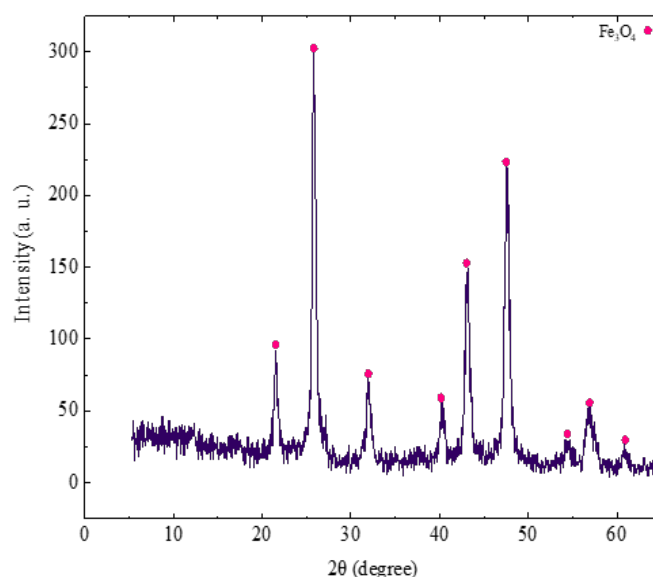
شکل ۳ نتایج آزمون XRD نمونه \text{Fe}_3\text{O}_4 سنتز شده Figure 3. XRD analysis results of the synthesized \text{Fe}_3\text{O}_4
