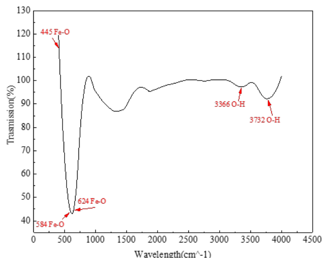
شکل ۲ نتایج آزمون FTIR نمونه \text{Fe}_3\text{O}_4 سنتز شده Figure 2. FTIR analysis results of \text{Fe}_3\text{O}_4 synthesized
