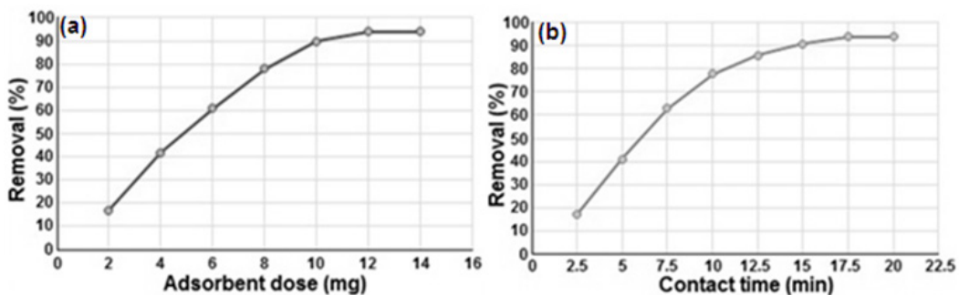
شکل ۶ a) تأثیرات مقدار جاذب \text{Fe}_3\text{O}_4@\text{SiO}_2 -EDTA بر روی میزان جذب یون های کادمیوم دوظرفیتی، b) اثرات زمان تماس جاذب بر روی جذب کادمیوم دوظرفیتی
