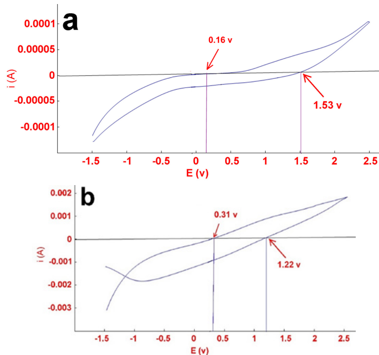
شکل ۱۰: نمودار CV نانوذرات ZnO-TDI و ZnO-PAni-Naph Figure 10: CV diagrams of a) ZnO-TDI and b) ZnO-PAni-Naph nanoparticles
