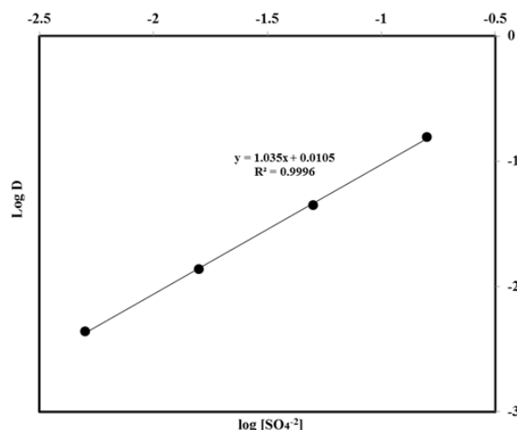
شکل ۸ اثر غلظت [SO_4^{2-}] بر استخراج سریم (IV). [غلظت یون فلزی در فاز آبی، 800 \text{ mg L}^{-1} ؛ استخراج‌کننده: 0.2 \text{ M} سیانکس ۹۲۱؛ دمای واکنش، 25 \pm 1^\circ \text{C} ؛ زمان تماس بین دو فاز، ۳ دقیقه] Fig. 8 Effect of SO_4^{2-} concentration on cerium (IV) extraction [Concentration of metal ions in the aqueous phase = 800 \text{ mg L}^{-1} ; Extractant concentration = 0.2 \text{ mol L}^{-1} Cyanex 921; pH=3; Reaction temperature = 25 \pm 1^\circ \text{C} ; Contact time between two phases = 3 min]
