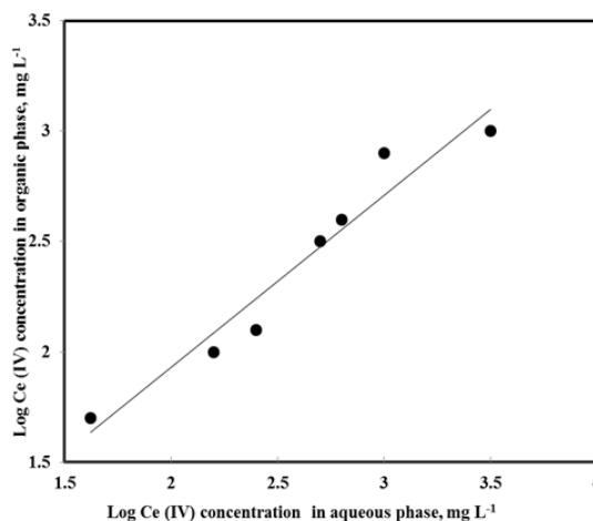
شکل ۶ تأثیر غلظت یون فلزی بر استخراج سریم (IV).
