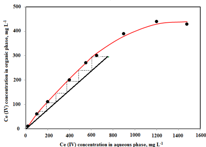
شکل ۹ هم‌دمای استخراج سریم (IV) با سیانکس ۹۲۱. Fig. 9 Cerium (IV) extraction isotherm with Cyanex 921
