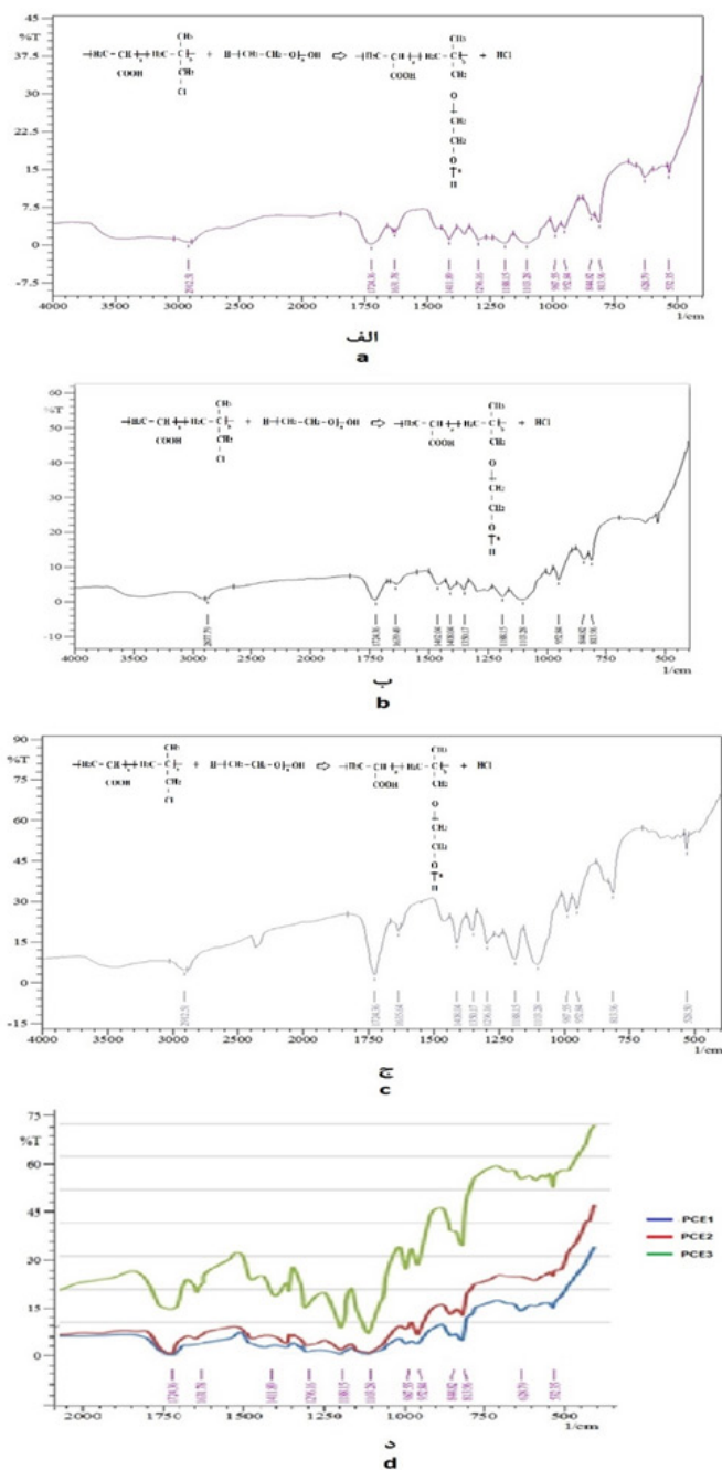
شکل ۴- طیف های FTIR پلی کربوکسیلات اتر سنتزی الف - طیف FTIR نمونه PCE ۱ ب- طیف FTIR نمونه PCE ۲ ج- طیف FTIR نمونه PCE ۳ د- مقایسه طیف های FTIR Fig- 4 FTIR spectra of Synthesized polycarboxylate ether a- FTIR spectrum of sample PCE1 b- FTIR spectrum of sample PCE2 c- FTIR spectrum of sample PCE3 d- Comparison of FTIR spectra
