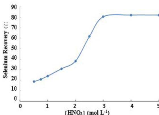
شکل ۲ تأثیر غلظت اسید نیتریک بر بازده فروشویی و بازیابی سلنیم [دما ۷۰ °C، نسبت جامد به مایع (W/V) ۰/۰۲، سرعت هم زدن ۲۰۰ rpm، زمان فروشویی ۴۵ دقیقه] Fig. 2 The effect of Nitric Acid concentration on leaching and recovery of selenium [Temperature 70°C, S/L 0.02 (w/v), stirring speed 200 rpm, leaching time 45min]
