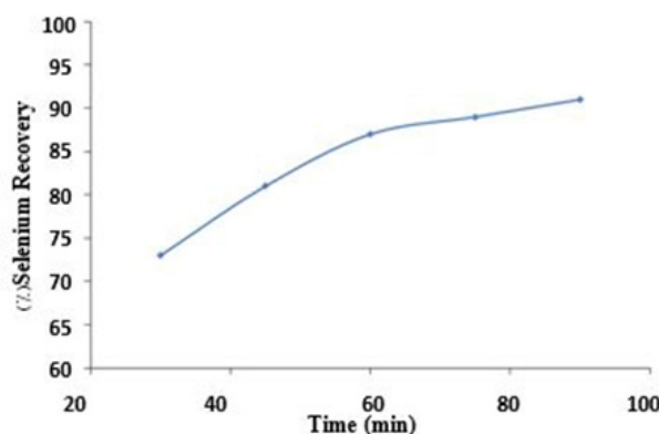
شکل ۴ سینتیک فروشویی و بازیابی سلنیم [غلظت اسید نیتریک 3 \text{ mol L}^{-1} ، دما 70^\circ\text{C} ، نسبت جامد به مایع 0.02 \text{ (W/V)} ، سرعت هم‌زدن 200 \text{ rpm} ] Fig. 4 Kinetics of leaching and recovery of selenium [Nitric acid concentration 3 \text{ mol L}^{-1} , Temp 70^\circ\text{C} , S/L 0.02 \text{ (w/v)} , stirring speed 200 \text{ rpm} ]
