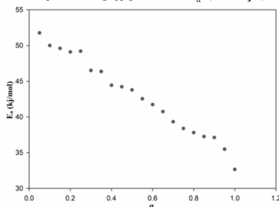
شکل ۷ وابستگی انرژی فعال سازی به مقدار تبدیل برای سامانه حامل HTPB-IPDI با کاتالیزور Fig. 7 Dependence of activation energy on conversion value for HTPB-IPDI binder system with catalyst
