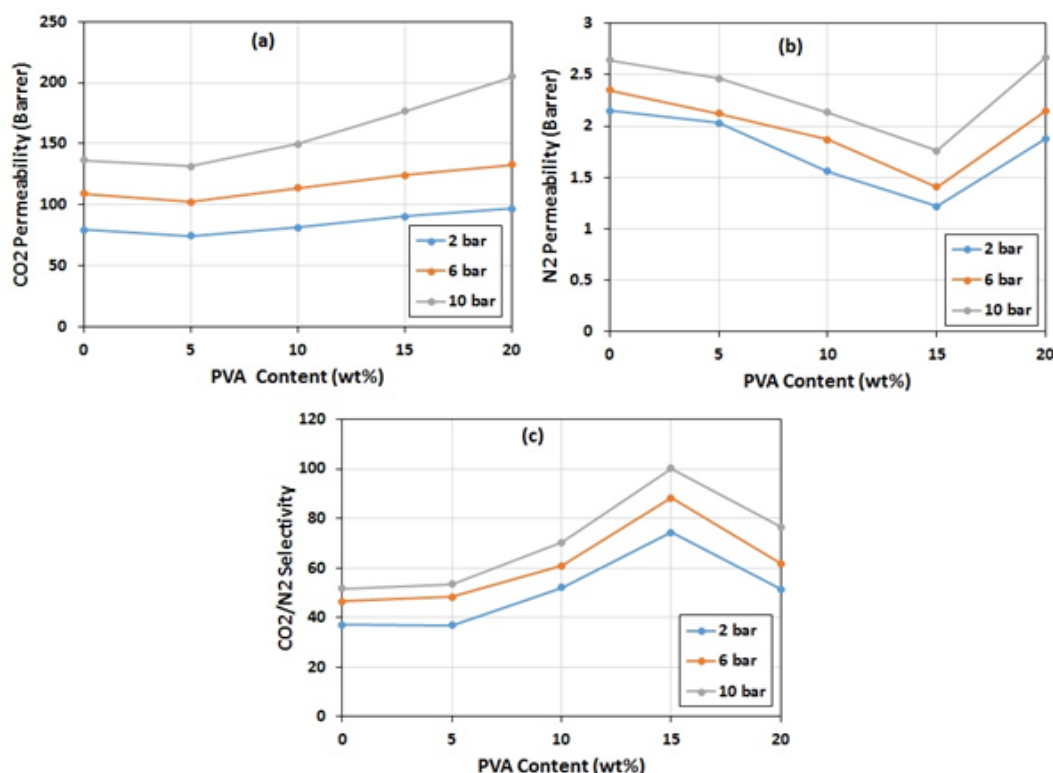
شکل ۶. اثر افزودن PVA و تغییرات فشار بر (a) تراوایی CO 2 ، (b) تراوایی N 2 و (c) انتخاب پذیری CO 2 /N 2 Figure 6. The effect of PVA content and pressure changes on (a) CO 2 permeability, (b) N 2 permeability, and (c) CO 2 /N 2 selectivity
