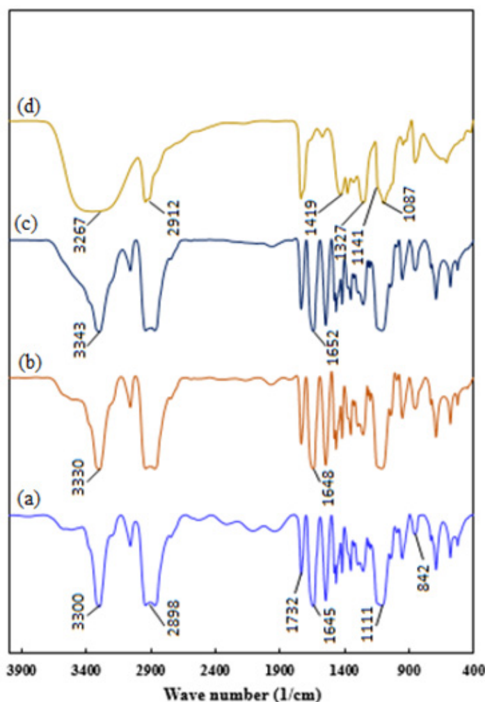
شکل ۱. نمودارهای FTIR غشاهای (a) Pebax، (b) Pebax/PVA ۵ درصد وزنی، (c) Pebax/PVA ۱۵ درصد وزنی، (d) PVA و PVA
