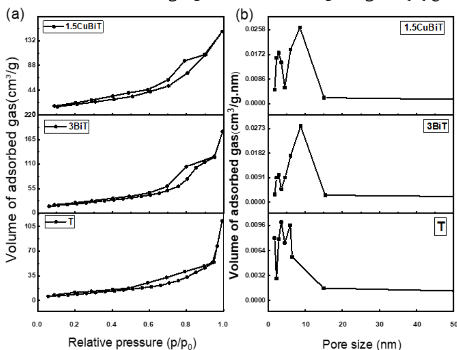
شکل ۵- (a) هم دمای جذب نیتروژن فوتوکاتالیست های T ، 3BiT و 1.5CuBiT در دمای ۷۷ کلوین (b) توزیع اندازه حفرات در فوتوکاتالیست های T ، 3BiT و 1.5CuBiT
