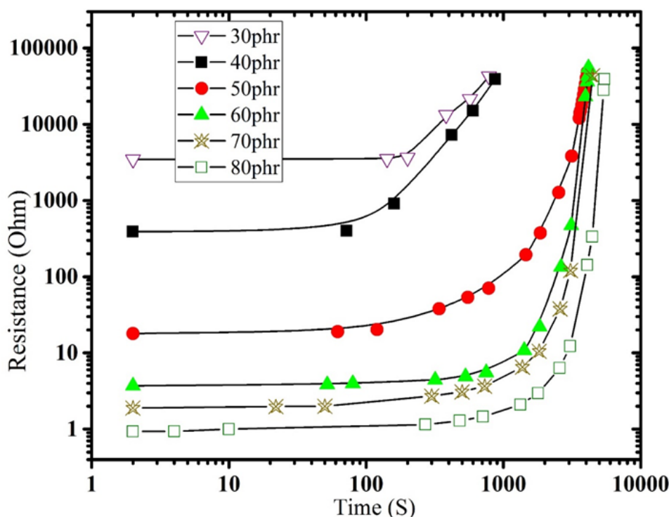
شکل ۴. تغییرات مقاومت الکتریکی نمونه‌های نیتریل/گرافیت حاوی ۲۰، ۳۰، ۴۰، ۵۰، ۶۰، ۷۰ و ۸۰ گرافیت بر حسب زمان تورم در حلال تولوئن در اولین غوطه‌وری در حلال
