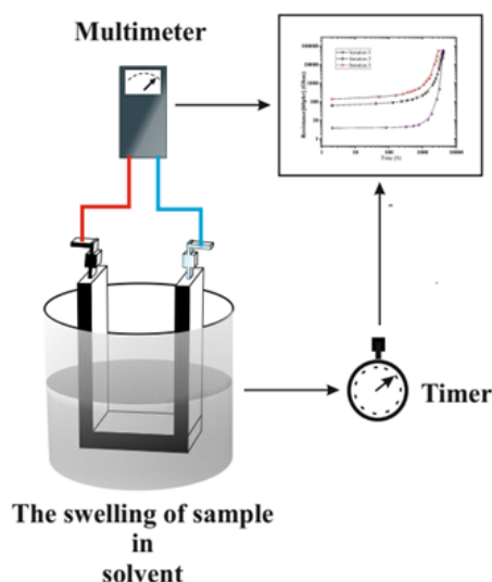
شکل ۲. طرح واره اندازه گیری مقاومت الکتریکی نمونه های کامپوزیت نیتریل/گرافیت بر حسب زمان تورم. Figure 2. Experimental set-up for measurement of electrical resistance of Nitrile/graphite rubber composite samples as function of swelling time.
