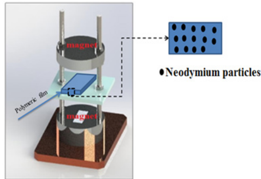
شکل ۱ طرح واره سامانه مورد استفاده برای ایجاد میدان مغناطیسی عمودی Figure 1 Scheme of the apparatus used to create orthogonal MF
