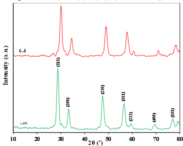
شکل ۲. طیف XRD نانوذرات CeO_2 (الف) و اکسید ترکیبی Ce_xZr_{1-x}O_2 (ب) Figure 2. XRD patterns of (a) CeO_2 and (b) Ce_xZr_{1-x}O_2 mixed oxide nanoparticles
