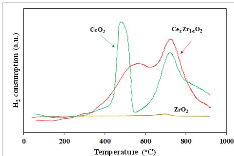
شکل ۵. منحنی \text{H}_2 -TPR مربوط به نانوذرات \text{CeO}_2 و \text{ZrO}_2 خالص و اکسید ترکیبی \text{Ce}_x\text{Zr}_{1-x}\text{O}_2 Figure 5. \text{H}_2 -TPR profiles for pure \text{CeO}_2 and \text{ZrO}_2 and \text{Ce}_x\text{Zr}_{1-x}\text{O}_2 mixed oxide nanoparticles
