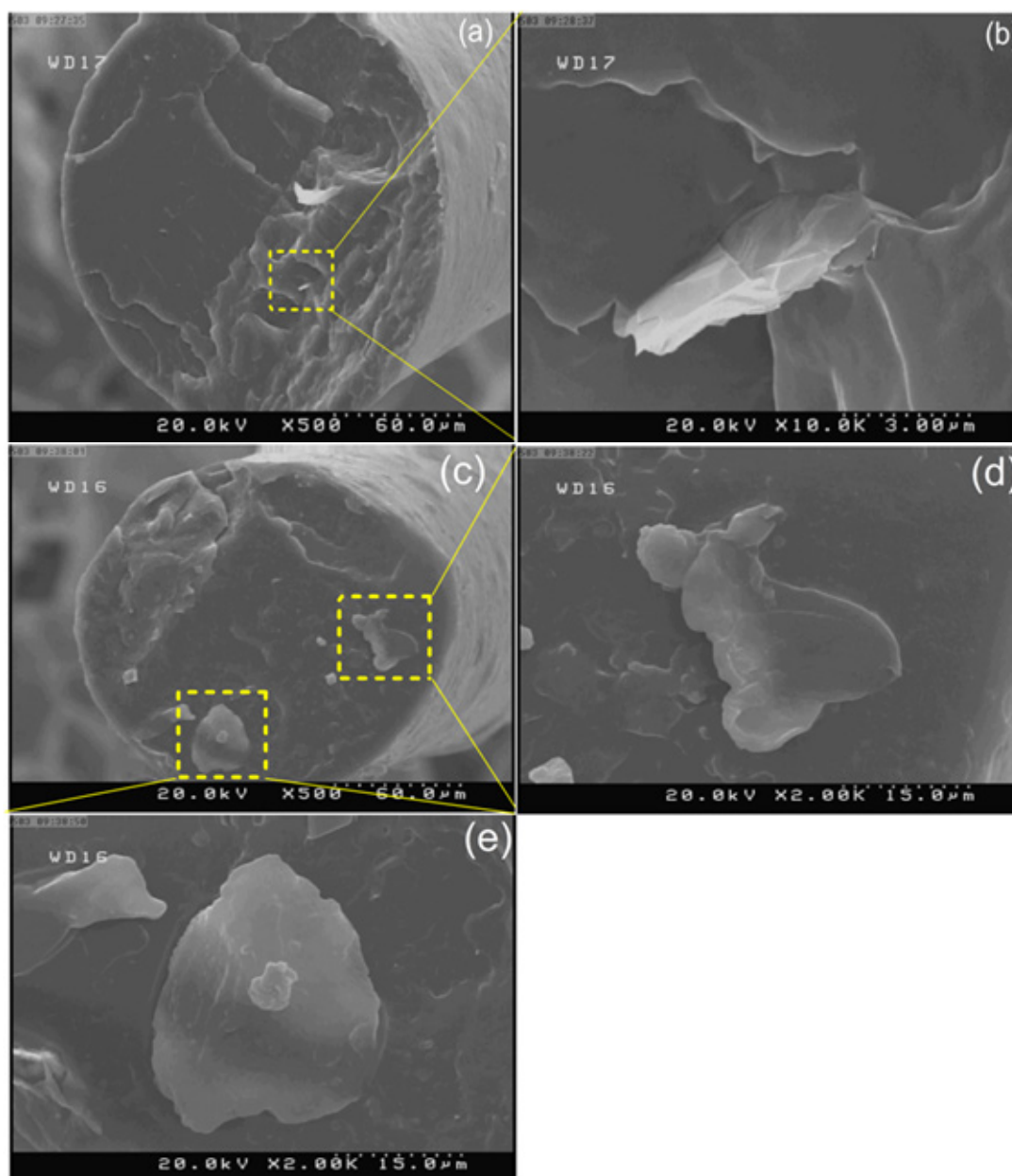
شکل ۶. تصاویر FESEM به دست آمده از سطح مقطع عرضی الیاف نانوکامپوزیت (a,b) PP/MA/G0.5 و (c-e) PP/G0.5 شکسته شده در نیتروژن مایع
