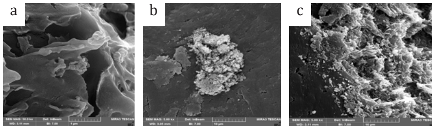
شکل ۳ تصویر (a) نانواکسیدگرافن، (b) نانوکامپوزیت GO/PMMA (GP2) با بزرگنمایی ۲۰۰۰ و (c) نانوکامپوزیت PMMA/GO (GP2) با بزرگنمایی ۵۰۰۰
