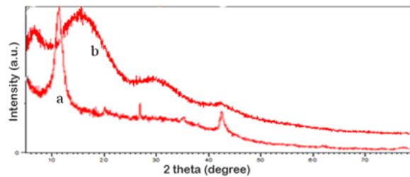
شکل ۲ طیف XRD (نانواکسیدگرافن، b) نانوکامپوزیت GO/PMMA (نمونه ۲) (a) نانوکامپوزیت GO/PMMA (GP2) nanocomposite
