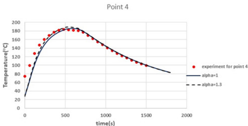
شکل ۶- تغییرات دمایی نقطه ای داخل تایر (مرز بلادر و لایه) در شرایط واقعی پخت بدست آمده از سیم گذاری و ثبت پروفایل دمایی (نقاط)، و شبیه سازی با مقادیر مختلف ضریب نفوذ حرارتی بلادر - خط \alpha=1 \times 10^{-7} و نقطه چین \alpha=1,3 \times 10^{-7}
