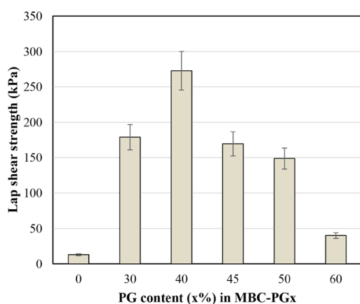
شکل ۸ استحکام برشی MBC30 خالص (X برابر با صفر) و آمیزه‌های MBC-PGx بر زیرآیند پلی‌استری بر حسب درصد PG Figure 8 Shear strength of pristine MBC30 (x equal to zero) and MBC-PGx blends on polyester substrate versus PG content
