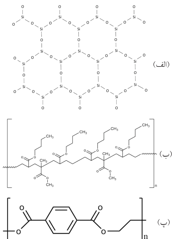
شکل ۶ ساختار شیمیایی (الف) شیشه، (ب) پلی(متیل متاکریلات - تصادفی - بوتیل اکریلات) و (پ) پلی(اتیلن ترفتالات)
