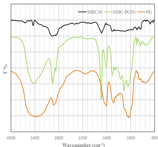
شکل ۴ طیف فروسرخ کاپلیمر اکریلیکی (MBC30)، صمغ پارسی (PG) و آلیاژ MBC-PG50
