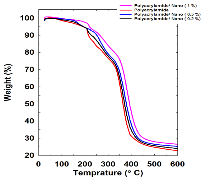
شکل ۵ نمودار TGA نانوکامپوزیت پلیمری با درصدیهای مختلف نانوسیلیکا Fig.5. TGA tests from nanocomposite with different nanosilica concentrations
