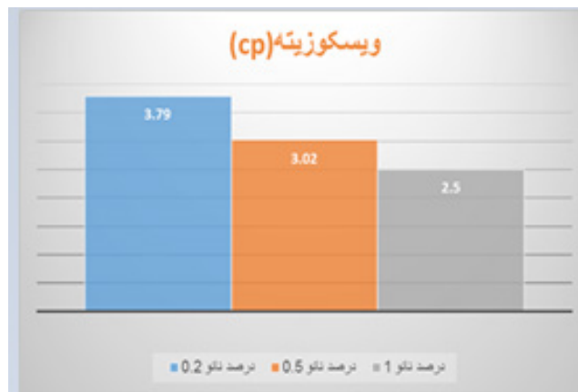
شکل ۸ نمودار آزمون گرانیروی برای محلول های نانوکامپوزیت پلیمری با درصدهای مختلف نانوسیلیکا در غلظت ppm ۱۰۰۰ آب سازند Fig.8. Viscosity results for nanocomposite solutions with different nanosilica concentrations and 1000 ppm water salinity
