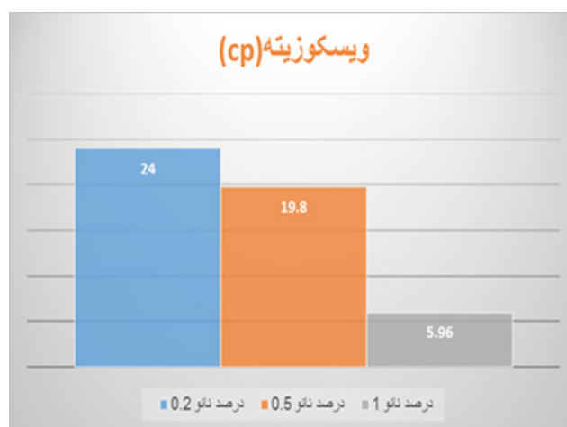
شکل ۹ نمودار آزمون گرانیروی برای محلول های نانوکامپوزیت پلیمری با درصدهای مختلف نانوسیلیکا در غلظت ppm ۲۰۰۰ آب سازند Fig.9. Viscosity results for nanocomposite solutions with different nanosilica concentrations and 2000 ppm water salinity
