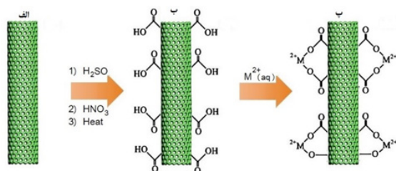
شکل ۳ سازوکار جذب یون های فلزی بر روی الف) نانولوله کربنی، ب) نانولوله کربنی اصلاح شده با \text{COOH} (پ) جذب فلزات توسط نانولوله کربنی اصلاح شده با \text{COOH} [۴۸]
