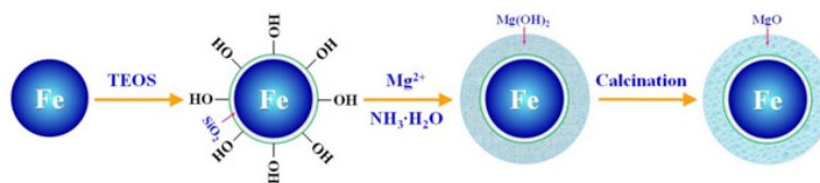
شکل ۶ طرحی از فرایند تشکیل نانوکامپوزیت Fe/MgO [۸۶].
