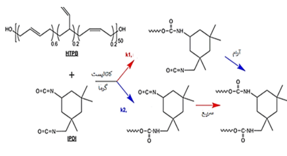
شکل ۲ طرح‌واره واکنش HTPB با IPDI [۳۶].
