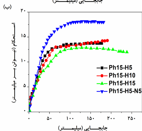
شکل ۳ نمودار نیرو بر حسب ازدیاد طول آزمون پوست کنی ۹۰ درجه برای نمونه های (الف) Gum، Ph-R5، Ph-R10 و Ph-R15 و (ب) Ph15-H5، Ph15-H10، Ph15-H15 و Ph15-H5-N5.
