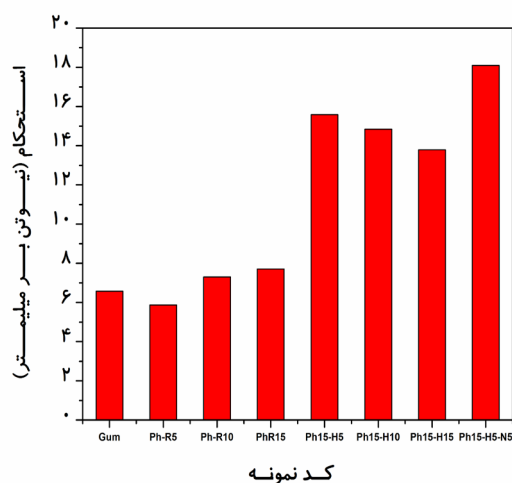
شکل ۴ نمودار میله ای نتایج آزمون پوست کنی ۹۰ درجه برای هشت نمونه بررسی شده.
