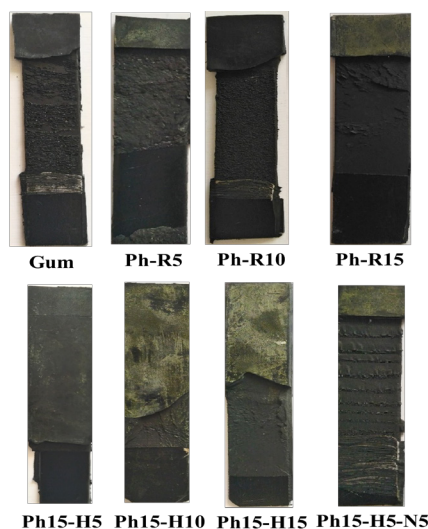
شکل ۵ تصاویر پس از آزمون پوست کنی ۹۰ درجه برای نمونه های مختلف
