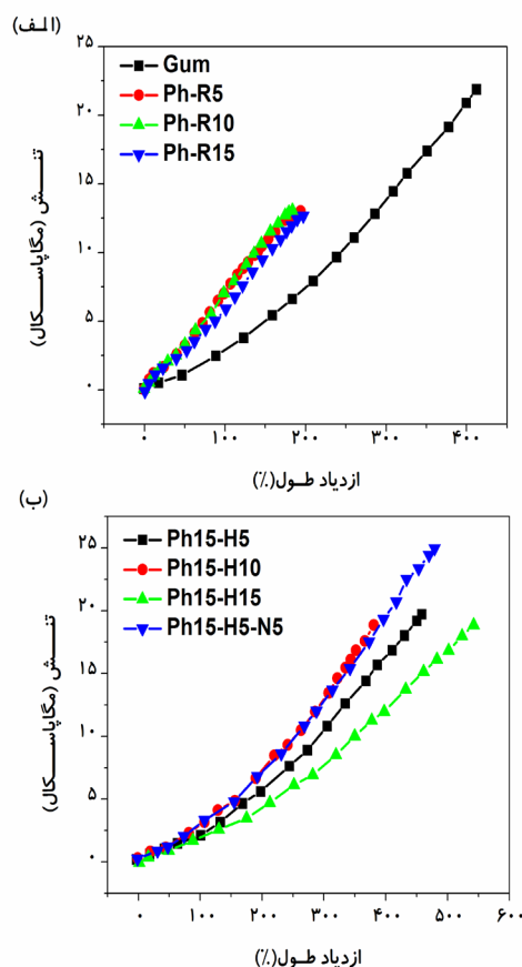
شکل ۲ نمودار تنش-کرنش نمونه های (الف) Gum، Ph-R5، Ph-R10، Ph-R15 و (ب) Ph15-H5، Ph15-H10، Ph15-H15 و Ph15-H5-N5
