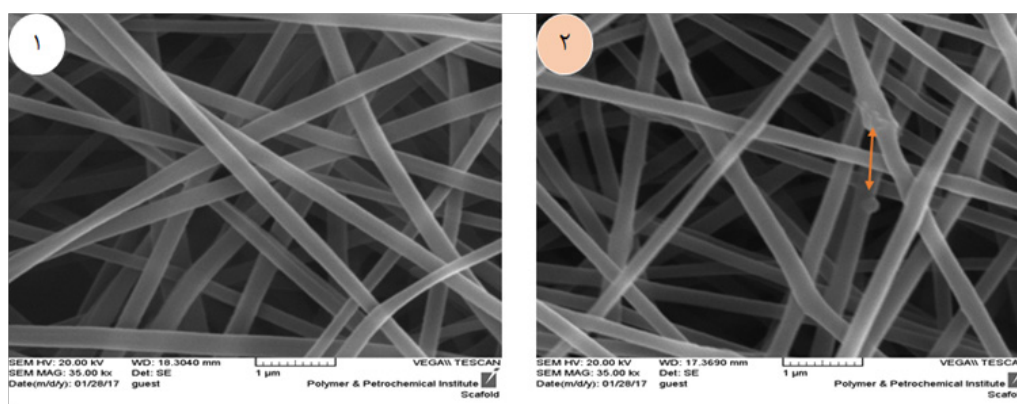
شکل ۴ تصویر میکروسکوپ الکترونی روبشی شامل (۱) نانوالیاف PVA و (۲) نقطه بهینه PVA / نانوببتونیت در بزرگ نمایی ۳۵.
