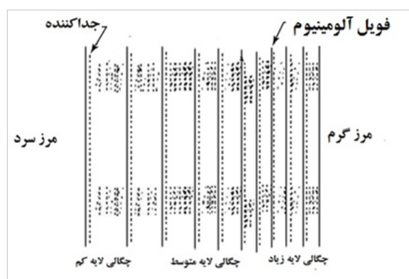
شکل ۱ ساختار و اجزای عایق چندلایه [۱]
