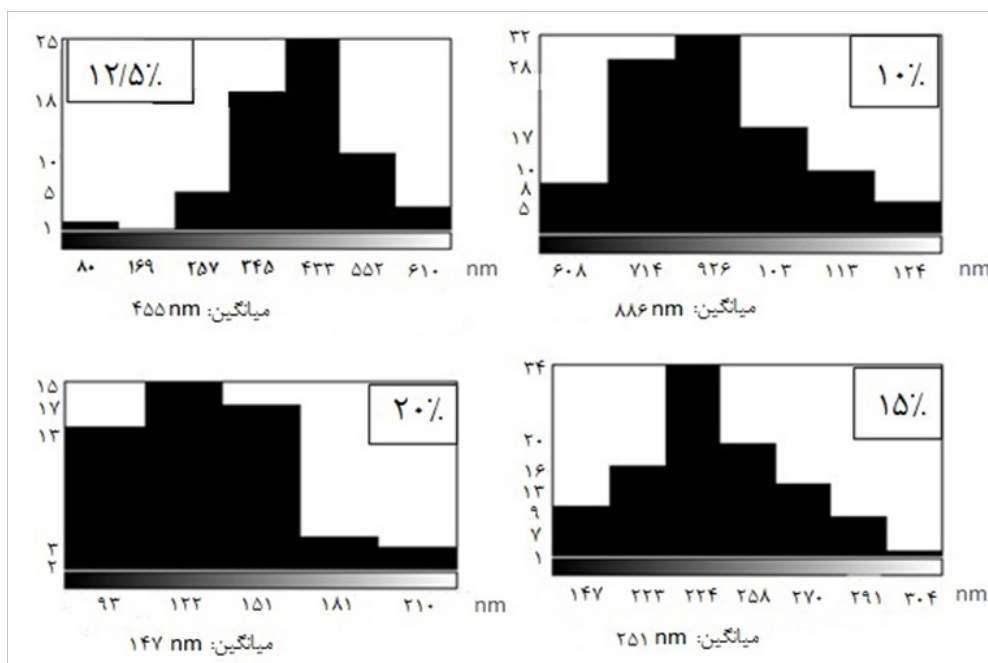
شکل ۷ توزیع میانگین قطر ذرات ابروژل تهیه شده از سل اولیه با درصدهای مختلف نووالاک
