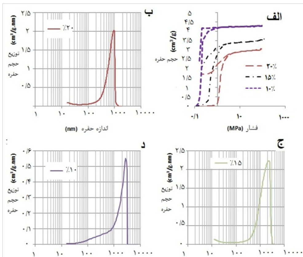
شکل ۸. بررسی ساختاری آبر متخلخل نووالاک به وسیله تخلخل سنج جیوه‌ای (الف) داده های خام تخلخل سنج جیوه‌ای نمونه‌ها، حجم تخلخل بر حسب فشار ب تا د) توزیع اندازه حفرات نمونه‌های به ترتیب ۲۰٪، ۱۵٪ و ۱۰٪ وزنی نووالاک در سل اولیه
