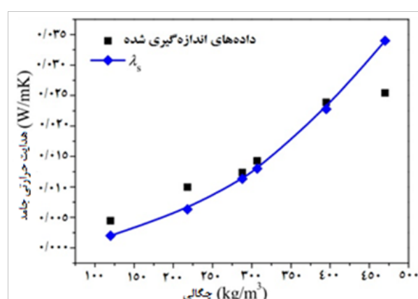
شکل ۳ تغییرات هدایت حرارتی جامد با تغییرات چگالی در ایروژل [۳].
