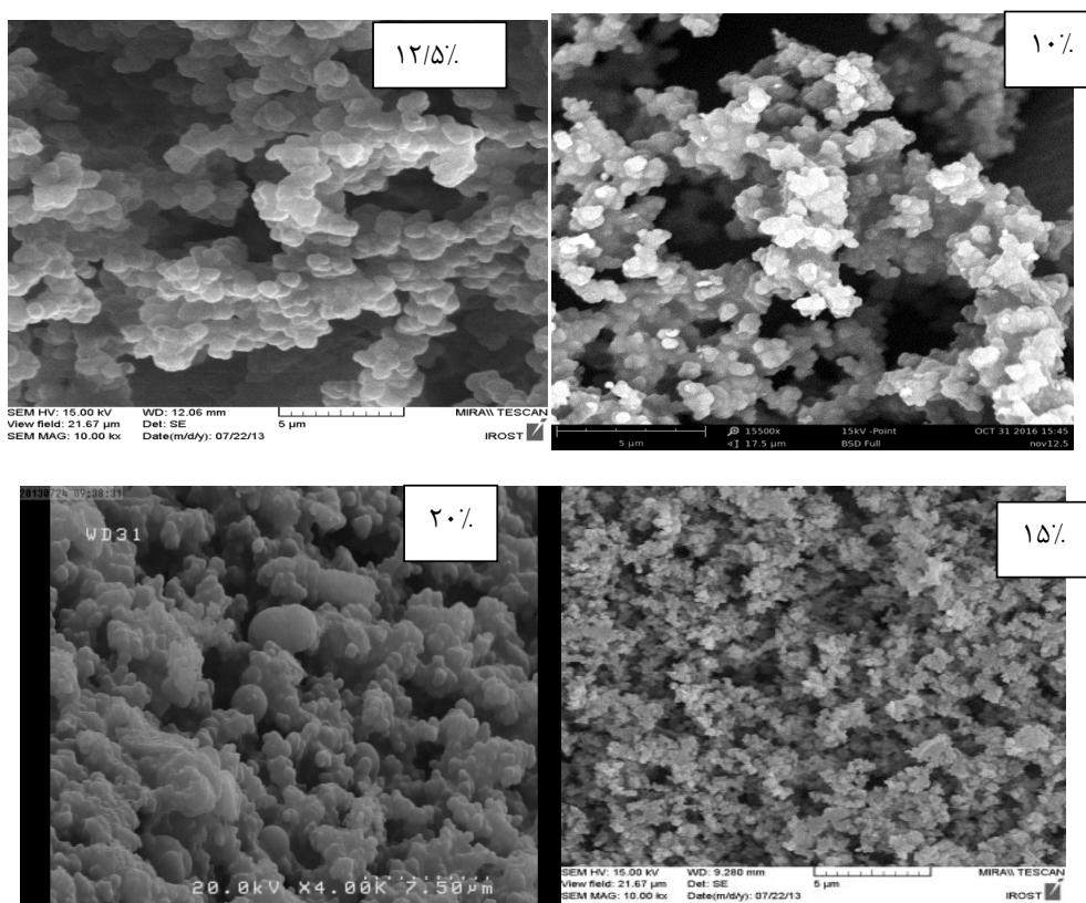
شکل ۶ ریز ساختار ابروژل نووالاک تهیه شده از درصدهای مختلف نووالاک در محلول سل اولیه
