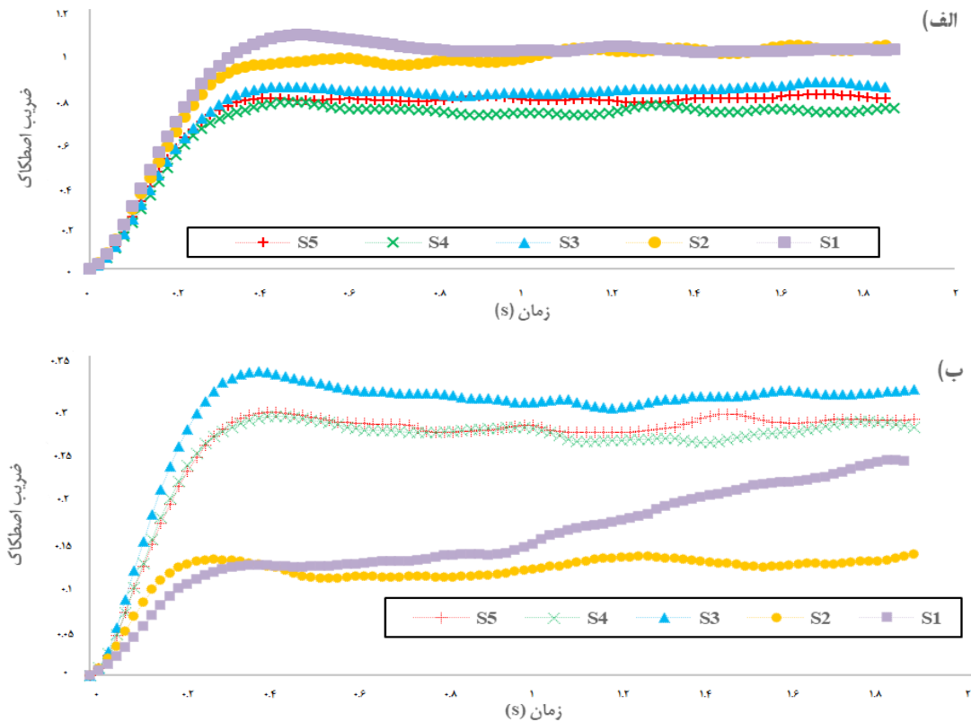
شكل ۳ تغييرات ضريب اصطكاك با شماره نمونه برداری به هنگام سُرش در مقابل سطوح مختلف بافت در (الف) شرایط خشک و (ب) روان کاری
