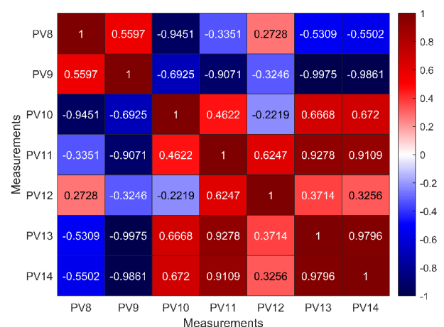
شکل ۸ تحلیل همبستگی متغیرهای اندازه‌گیری
