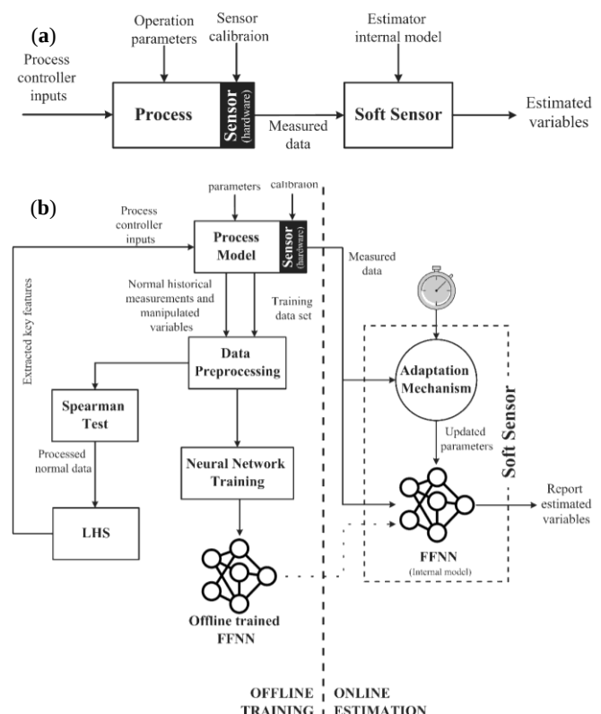
شکل ۶ (a) نحوه به‌کارگیری حسگر نرم در فرایند؛ (b) ساختار حسگر نرم طراحی شده و رویه آموزش برون خط حسگر نرم و به‌کارگیری برخط آن
