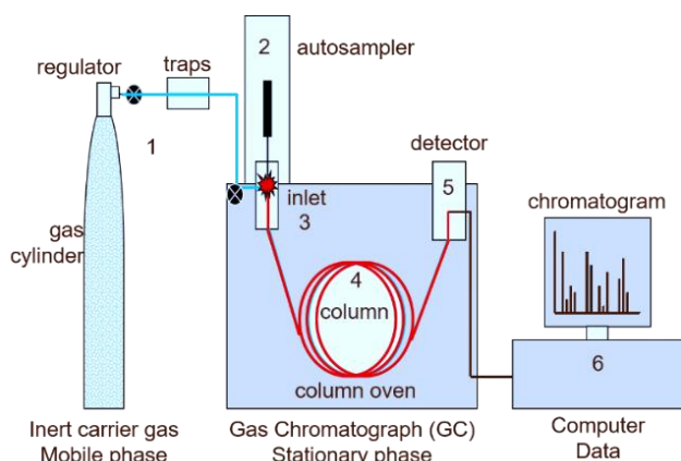
شکل ۱ مراحل اندازه‌گیری دستگاه کروماتوگرافی گازی [۵]
