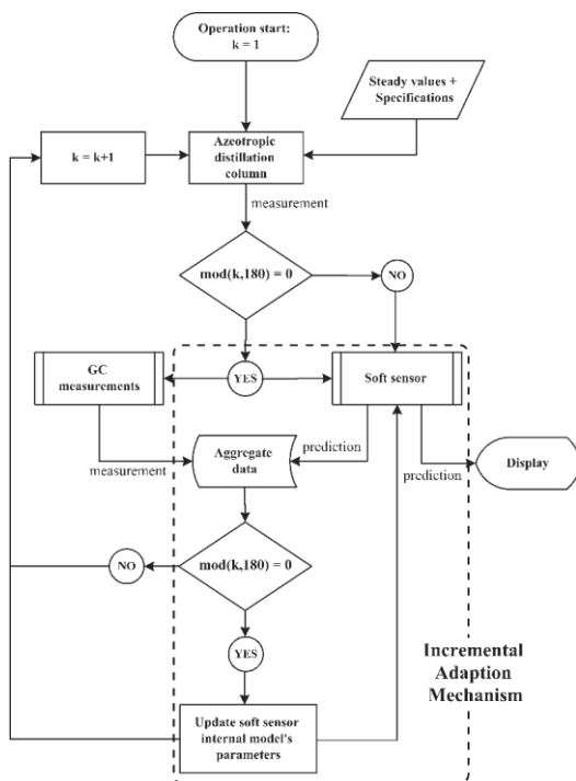
شکل ۷ الگوریتم سازوکار تطبیقی تدریجی حسگر نرم
