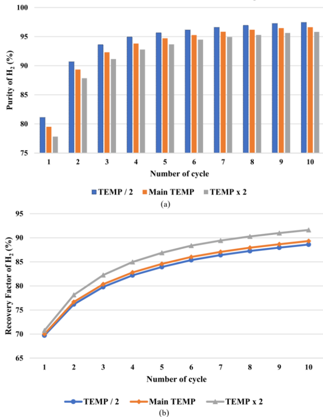
شکل ۸ تأثیر دما بر روی (الف) خلوص و (ب) ضریب بازیافت هیدروژن
