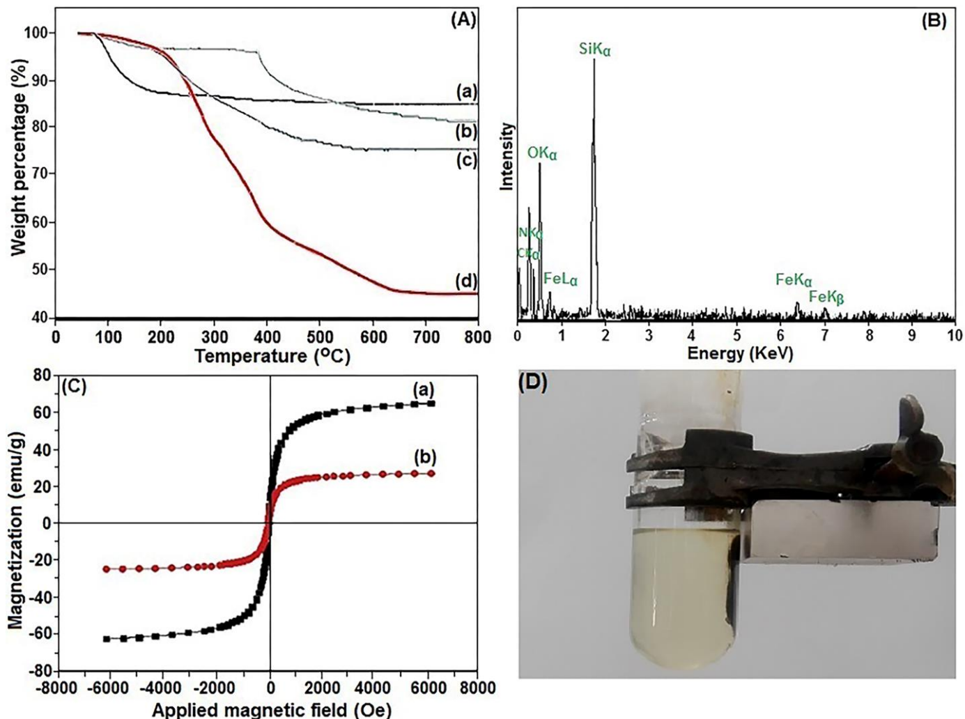
شکل ۵ (A) نمودارهای آزمون گرمایزن سنجی (TGA) برای (a) نانوذرات \text{Fe}_3\text{O}_4/\text{SiO}_2 ، (b) \text{Fe}_3\text{O}_4/\text{SiO}_2\text{-Cl} ، (c) \text{Fe}_3\text{O}_4/\text{SiO}_2\text{-TCT} و (d) \text{Fe}_3\text{O}_4/\text{SiO}_2\text{-TCT-PVA} . (B) نمودار پراش انرژی پرتو ایکس (EDX) نانوذرات \text{Fe}_3\text{O}_4/\text{SiO}_2\text{-TCT-PVA} . (C) نمودار مغناطیس سنج نمونه مرتعش (VSM) نانوذرات (a) \text{Fe}_3\text{O}_4 و (b) \text{Fe}_3\text{O}_4/\text{SiO}_2\text{-TCT-PVA} در دمای ۳۰۰ K و (D) توانایی بازیابی جاذب با استفاده از آهنربای مغناطیسی
