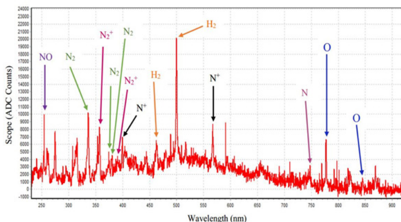
شکل ۳ طیفسنجی گسیل نوری از پلاسمای جرقه لغزان
