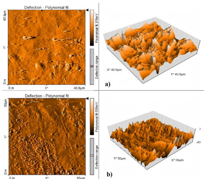
شکل ۱۱ (a) تصویر نمونه کنترل با میکروسکوپ نیروی اتمی و (b) تصویر نمونه اصلاح شده با میکروسکوپ نیروی اتمی Figure 11 a) Image of the control sample with Atomic Force Microscopy and b) Image of the modified sample with Atomic Force Microscopy
