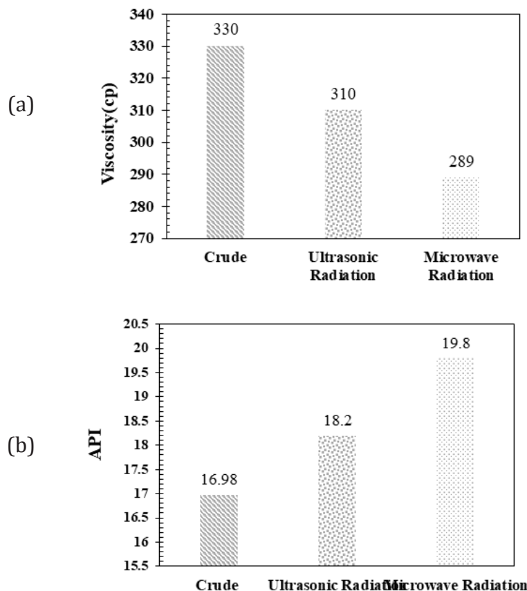
شکل ۲. الف) گرانی و ب) درجه API نفت خام و نفت تحت تابش امواج فراصوت و ماکروویو Figure 2. a) Viscosity and b) API gravity of crude oil and oil under ultrasonic and microwave radiation
