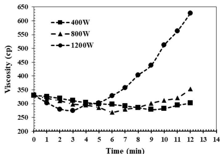
شکل ۳. تغییرات گرانی و نفت تحت تابش امواج ماکروویو در زمان و توان‌های مختلف Figure 3. Changes in oil viscosity under microwave radiation at different times and power levels
