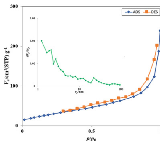
شکل ۷ آزمون جذب و واجذب نیتروژن و توزیع اندازه حفرات نمونه GAE Figure 7 \text{N}_2 adsorption/desorption and pore size distribution of GAE
