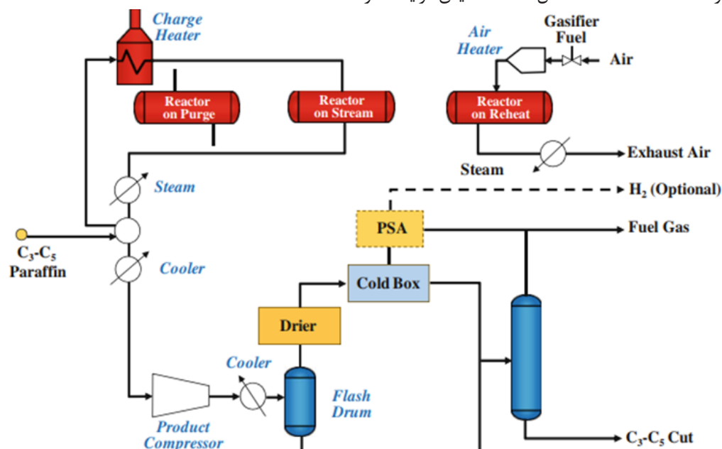
شکل ۴ نمودار جریان فرایند Catofin [۳] Figure 4. Catofin process flow diagram [3]
