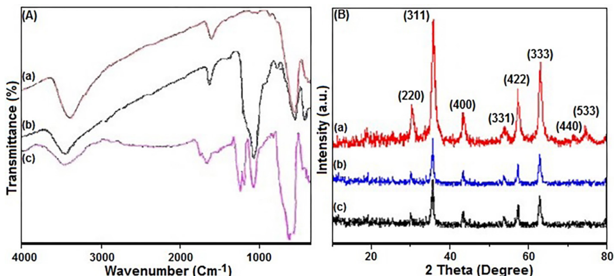
شکل ۱ (A) طیف FT-IR نانوذرات \text{MnFe}_2\text{O}_4 (a)، \text{MnFe}_2\text{O}_4@\text{SiO}_2 (b) و \text{MnFe}_2\text{O}_4@\text{SiO}_2@\text{PMIDA} (c) و (B) خصوصیات پراش پرتوی ایکس برای نانوذرات \text{MnFe}_2\text{O}_4 (a)، \text{MnFe}_2\text{O}_4@\text{SiO}_2 (b) و \text{MnFe}_2\text{O}_4@\text{SiO}_2@\text{PMIDA} (c) Figure 1. (A) FT-IR spectra of (a) \text{MnFe}_2\text{O}_4 , (b) \text{MnFe}_2\text{O}_4@\text{SiO}_2 and (c) \text{MnFe}_2\text{O}_4@\text{SiO}_2@\text{PMIDA} nanoparticles and (B) X-ray diffraction characteristics for (a) \text{MnFe}_2\text{O}_4 , (b) \text{MnFe}_2\text{O}_4@\text{SiO}_2 and (c) \text{MnFe}_2\text{O}_4@\text{SiO}_2@\text{PMIDA}
