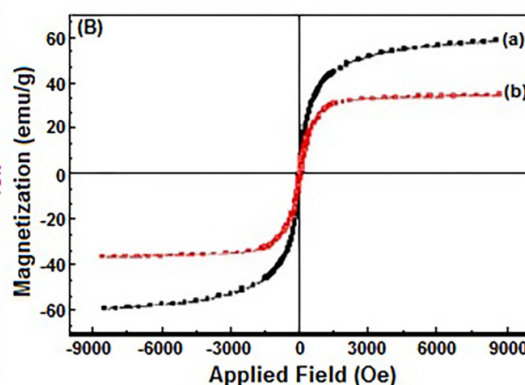
شکل ۳ (A) الگوی آزمون توزین حرارتی \text{MnFe}_2\text{O}_4@\text{SiO}_2@\text{PMIDA} . (B) تصویر VSM نانوذرات (a) \text{MnFe}_2\text{O}_4 و (b) \text{SiO}_2@\text{PMIDA}
