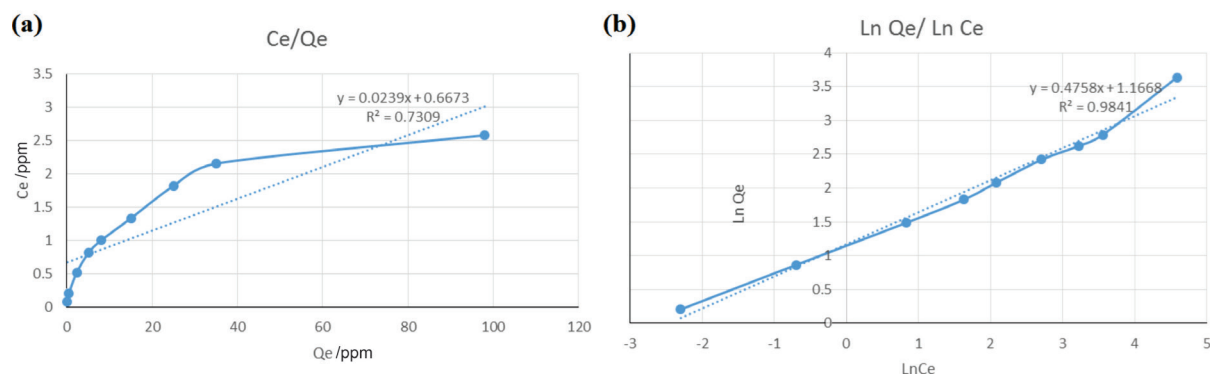
شکل ۷ (a) هم‌دمای جذب لانگمویر و (b) هم‌دمای جذب فرندلیچ یون‌های \text{Cr(VI)} بر روی جاذب Figure 7. a) Langmuir adsorption isotherm and b) Freundlich adsorption isotherm of \text{Cr(VI)} ions on the adsorbent
