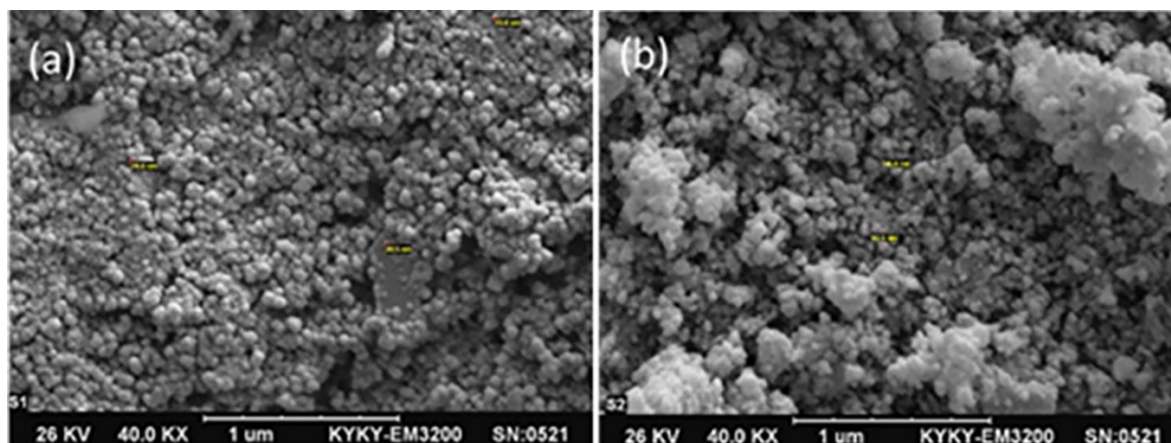
شکل ۲ تصویر SEM نانوذرات (a) \text{MnFe}_2\text{O}_4 و (b) \text{MnFe}_2\text{O}_4@\text{SiO}_2@\text{PMIDA} Figure 2. SEM image of (a) \text{MnFe}_2\text{O}_4 and (b) \text{MnFe}_2\text{O}_4@\text{SiO}_2@\text{PMIDA} nanoparticles
