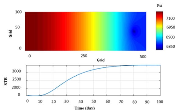
شکل ۹ تغییرات فشار مخزن و دبی چاه در حالتی که چاه از منبع تولید موج ۱۸۰۰ فوت فاصله دارد
