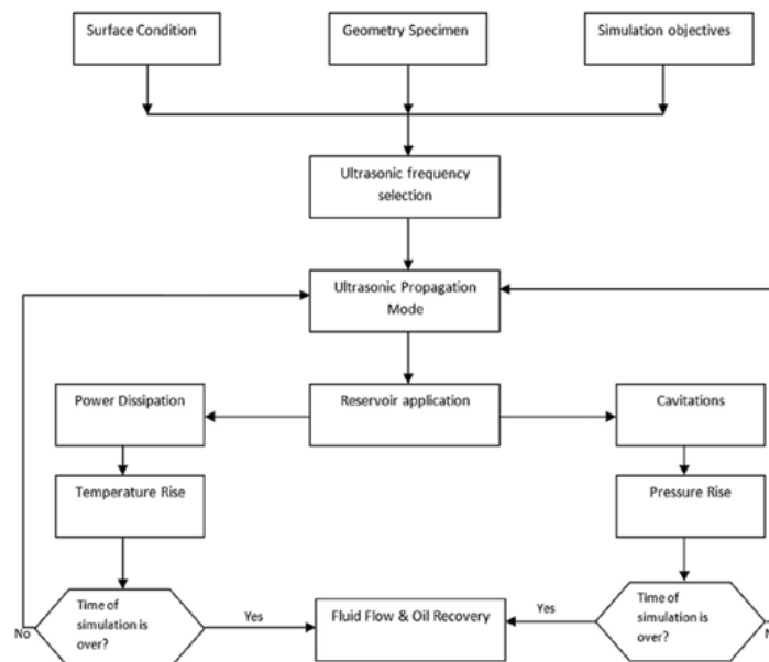
شکل ۲. فلوچارت مورد استفاده در شبیه سازی فرایند Figure 2. The used flowchart in simulation of the process.
