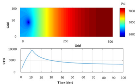
شکل ۸ تغییرات فشار مخزن و دبی چاه در حالتی که چاه از منبع تولید موج ۲۰۰ فوت فاصله دارد
