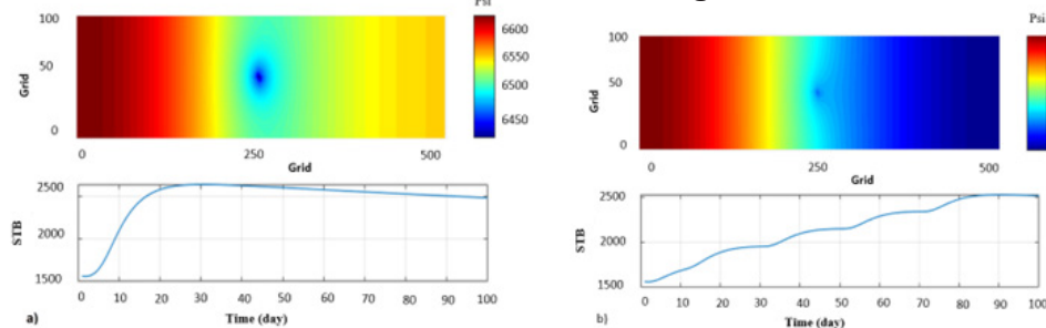
شکل ۷ تغییرات فشار مخزن و دبی چاه برای نحوه اعمال موج به مدت ۵ روز در دو حالت: الف) پیوسته و ب) پالسی Figure 7 Changes in reservoir pressure and well flow rate for wave apply states with 5 days in two modes: a) continuous and b) pulsed
