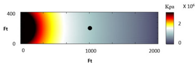
شکل ۳ توزیع فشار صوتی در مخزن با فرکانس ۲۰ کیلوهرتز و توان ۵ کیلووات Figure 3. Sonic Pressure distribution in the reservoir with frequency of 20 kHz and power of 5 Kw.
