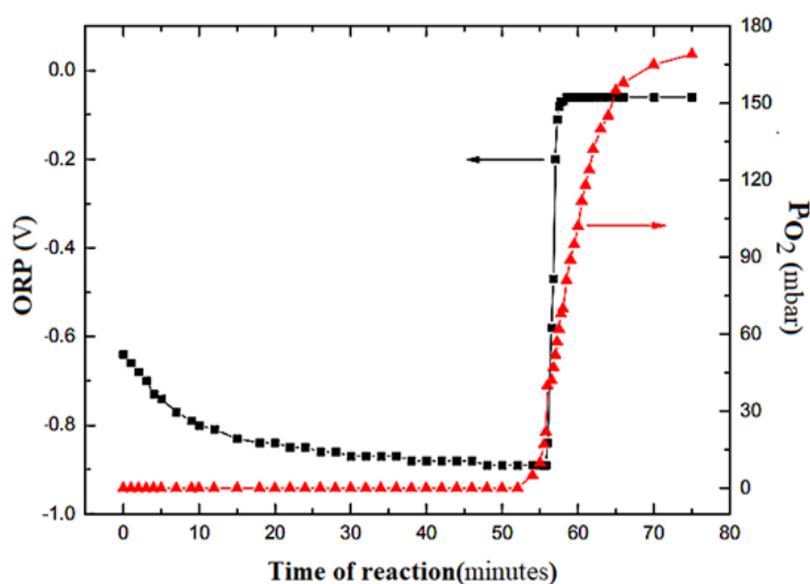
شکل ۸ نمودار پتانسیل اکسایش-کاهش (ORP) (■) و اکسیژن محلول (DO) (▲) بر حسب زمان، در آزمایش انجام شده با روش اکسیداسیون محلول و با پیش‌ماده‌های NaOH و FeSO_4 ، توسط انجینا (Encina) و همکاران [۲۰]
