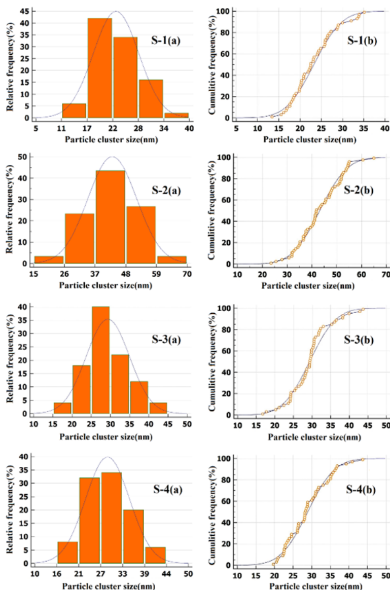
شکل ۵ نمودار توزیع اندازه‌ی مجموعه‌ذرات در نمونه‌ها، (a) درصد فراوانی نسبی، (b) درصد فراوانی تجمعی Figure 5. The plot of particle cluster size distribution in samples: (a) Relative frequency, (b) Cumulative frequency
