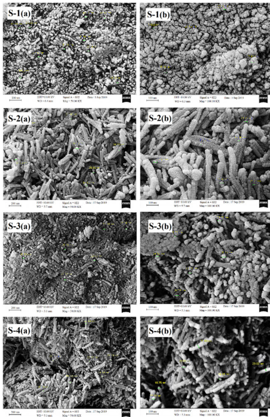
شکل ۴ تصاویر میکروسکوپ الکترونی بویشی از نمونه‌ها با بزرگ‌نمایی (a) ۵۰۰۰ و (b) ۱۰۰۰۰ برای Figure 4. The pictures of field emission scanning electron microscopy (FESEM) from samples with magnification of (a) 50000 and (b) 10000X
