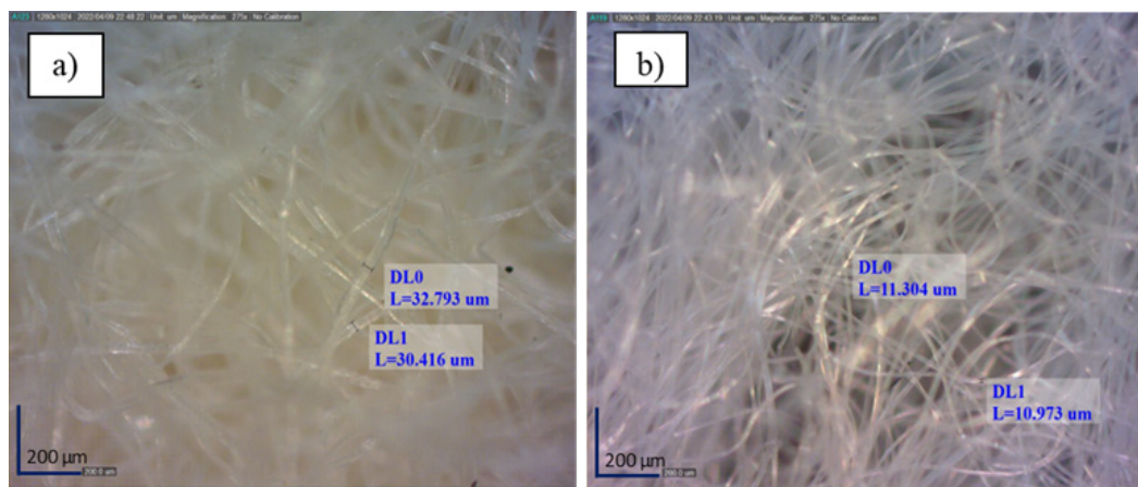
شکل ۵ تصاویر میکروسکوپ نوری از الف) نم‌پنبه‌ای و ب) نم‌پلی‌استری
