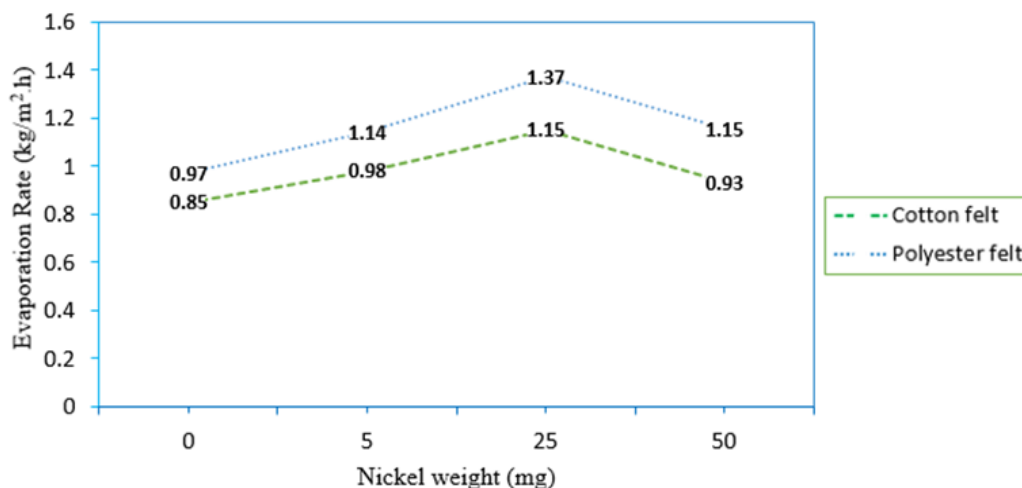
شکل ۷ نمودار نرخ تبخیر بر اساس مقدار جاذب فوتوترمال نیکل Figure 7. The plot of evaporation rate vs. nickel photothermal absorber weight
