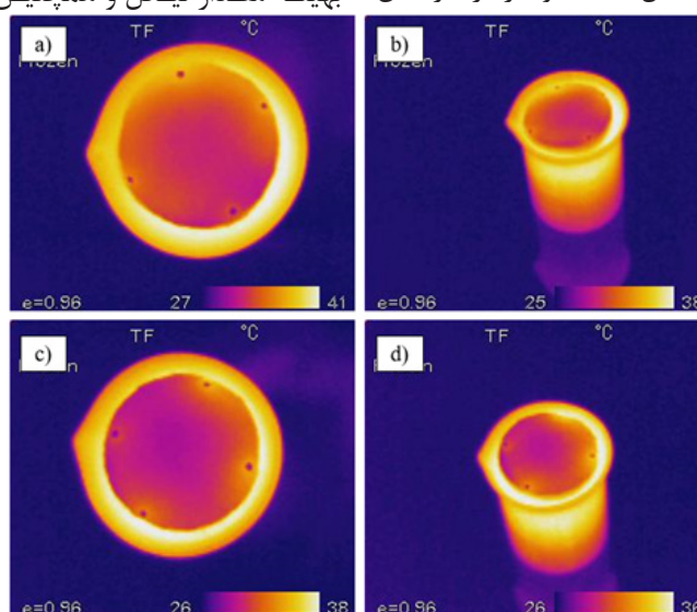
شکل ۸ تصویر دوربین حرارتی الف و ب) از بالا و کنار سامانه با نم‌د پنبه‌ای و ج و د) از بالا و کنار سامانه برای نم‌د پلی‌استری Figure 8. Thermographic camera images, a and b) top and side views of the cotton felt system and c and d) Top and side views of the polyester felt system
