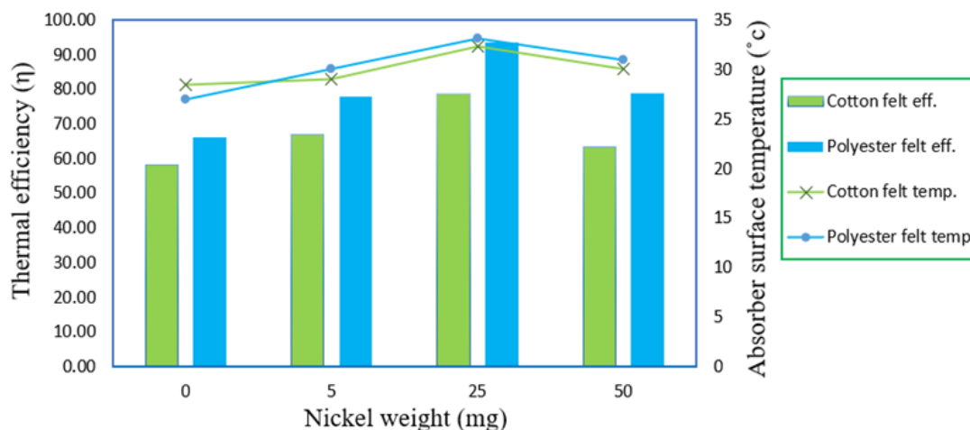
شکل ۹ نمودار بازده حرارتی و دمای سطح بر اساس مقدار جاذب فتوترمال گرافیت/نیکل برای نمدهای پنبه‌ای و پلی‌استری Figure 9. Thermal efficiency and surface temperature vs. graphite/nickel photothermal absorbers for cotton and polyester felts
