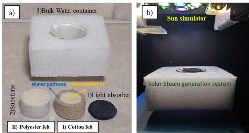
شکل ۲ الف) تصویر اجزای سازنده سامانه خورشیدی تولید بخار، شامل (۱) جاذب فتوترمال، (۲) زیرلایه به صورت فوم پلی‌پورتان پیچیده شده در نمد و (۳) مخزن توده آب. زیرلایه همراه با (I) نمد پنبه‌ای و (II) نمد پلی‌استری. ب) تصویر سامانه زیر تابش نور شبیه‌ساز خورشیدی Figure 2. a) Illustration of the solar steam generation system, including the 1) photothermal absorber, 2) polyurethane foam covered by felt as a substrate, and 3) bulk water mass container. A substrate with I) cotton felt and II) with polyester. b) Image of the system under the light of the solar simulator
