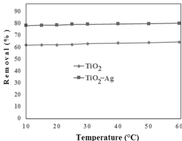
شکل (۷): بررسی اثر دما بر روی حذف متریبوزین Figure (7): Investigating the effect of temperature on metribuzin removal
