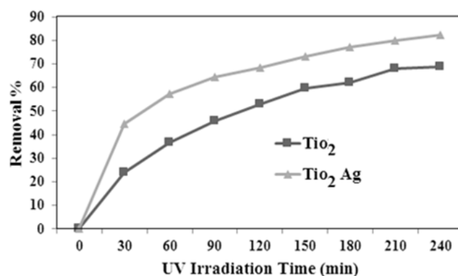
شکل (۵): تاثیر زمان واکنش بر حذف فتوکاتالیستی متریبوزین توسط کاتالیست‌های سنتز شده برای غلظت اولیه ۱۰ میلی گرم بر لیتر متریبوزین و دمای ۲۵ درجه سانتی گراد
