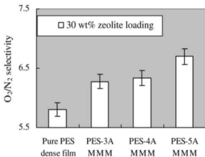
شکل ۵ تأثیر اندازه حفره های زئولیت در گزینش پذیری غشای شبکه آمیخته [۷۵] Fig. 5 effect of different pore sizes of zeolite on O 2 /N 2 selectivity of mixed matrix membranes [75]
