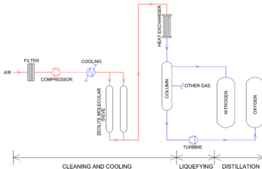
شکل ۱ طرحواره فرایند تقطیر برودتی [۱۵]
