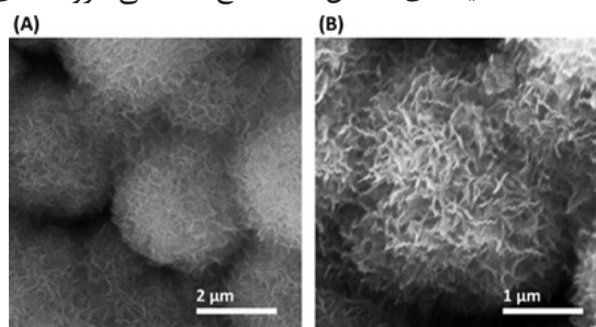
شکل ۳ تصاویر SEM نانوذرات معدنی rHAp در بزرگ‌نمایی کم (A) و بزرگ‌نمایی زیاد (B) بعد از ۳۰ روز خواباندن در محلول SBF. Fig. 3. SEM images of rHAp inorganic nanoparticles. at low magnification (A) and high magnification (B) after 30 days of incubation in SBF solution.
