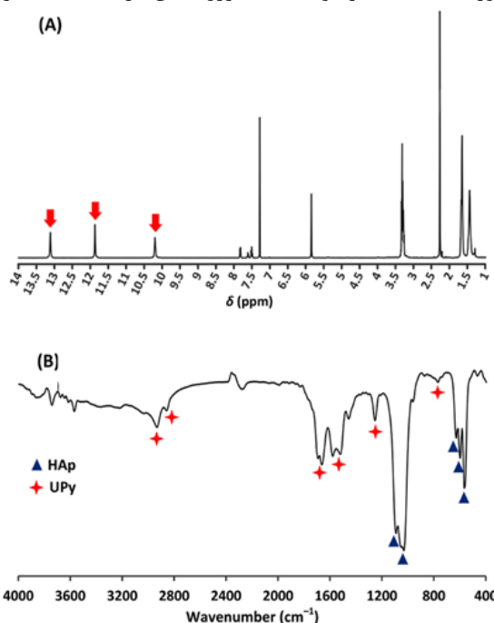
شکل ۴ (A) طیف ^1H\text{ NMR} گروه UPy در کلروفرم دوتره؛ (B) طیف FTIR نانوذرات معدنی rHAp اصلاح‌سطحی شده. Fig. 4. (A) ^1H\text{ NMR} spectrum of UPy group in deuteriochloroform; (B) FTIR spectrum of surface-modified rHAp inorganic nanoparticles.
