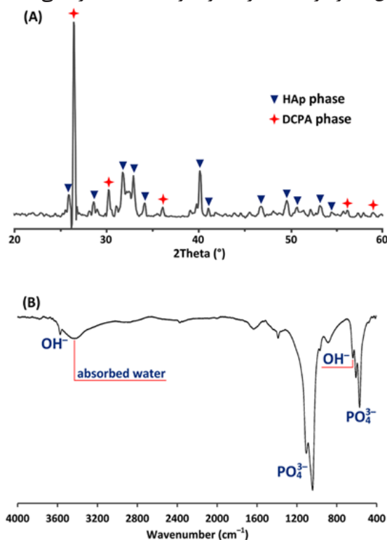
شکل ۱ طیف ۱ طیف XRD (A) و طیف FTIR نانوذرات معدنی rHAp. Fig. 1. XRD spectrum (A) and FTIR spectrum (B) of rHAp inorganic nanoparticles.
