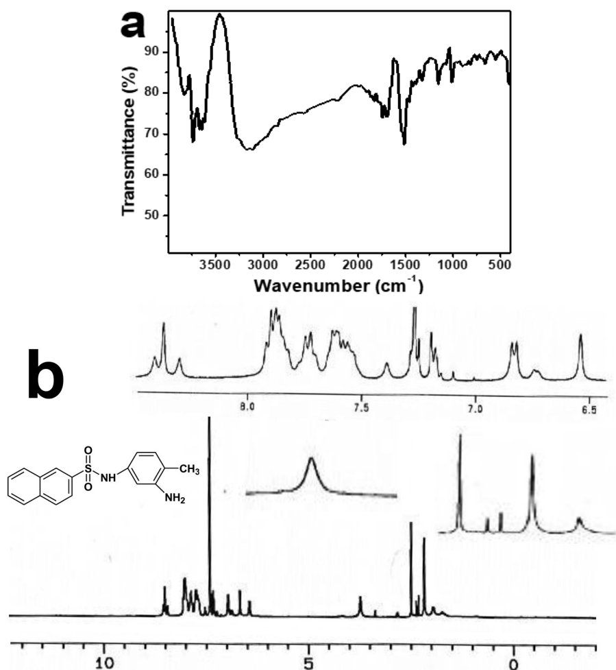
شکل ۳: طیف‌های: (a) FT-IR و (b) ^1\text{H NMR} ترکیب N-(۳-آمینو-۴-متیل فنیل)نفتالن-۲-سولفونامید Figure 3: FT-IR (a) and ^1\text{H NMR} (b) spectra of N-(3-amino-4-methylphenyl)naphthalene-2-sulfonamide
