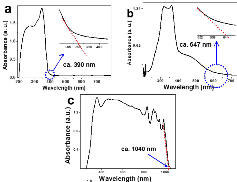
شکل ۹: طیف UV-Vis نانوذرات ZnO خالص، a) ZnO-TDI و b) ZnO-PAni-Naph و c) ZnO-PAni-Naph Figure 9: UV-Vis spectra of a) bare ZnO, b) ZnO-TDI and c) ZnO-PAni-Naph nanoparticles
