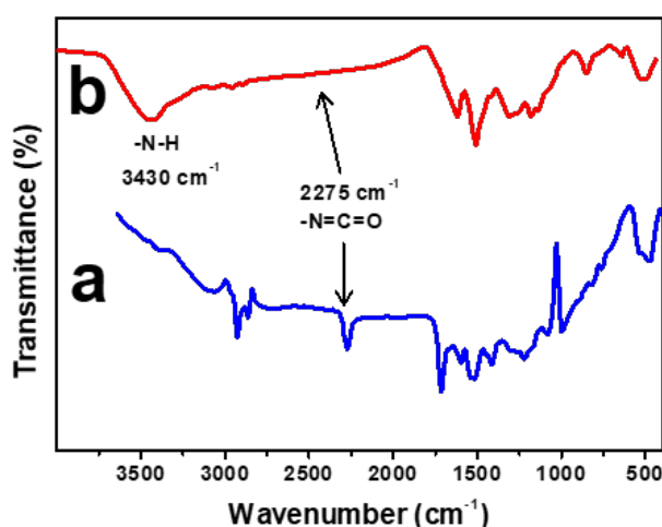
شکل ۶: طیف FT-IR نانوذرات a) ZnO-TDI و b) ZnO-PAni-Naph Figure 6: FT-IR spectra of a) ZnO-TDI and b) ZnO-PAni-Naph nanoparticles
