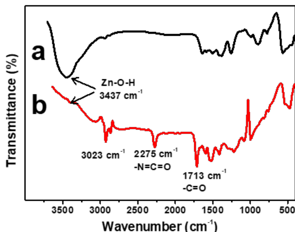
شکل ۵: طیف FT-IR نانوذرات a) ZnO خالص و b) ZnO-TDI Figure 5: FT-IR spectra of a) bare ZnO and b) ZnO-TDI nanoparticles
