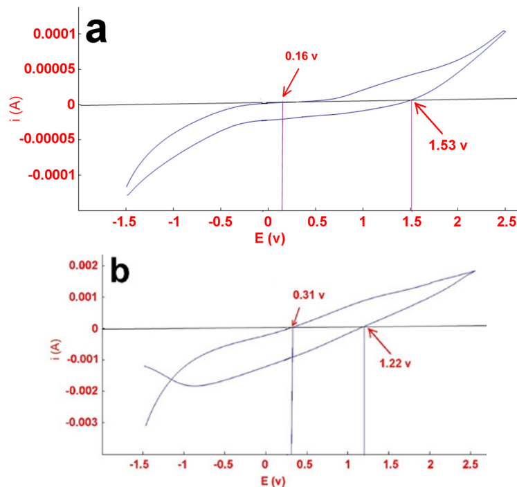
شکل ۱۰: نمودار CV نانوذرات ZnO-TDI و a) ZnO-TDI و b) ZnO-PAni-Naph Figure 10: CV diagrams of a) ZnO-TDI and b) ZnO-PAni-Naph nanoparticles
