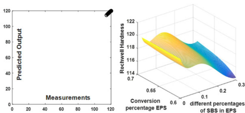
شکل ۱۴: عملکرد یاد آوری و تعمیم شبکه MLP برای تست مقدار سختی پلیمر در درصد تبدیل‌های مختلف EPS و درصد‌های مختلف SBS/
