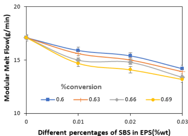
شکل ۳: نتایج آزمون شاخص جریان مذاب در درصد‌های مختلف SBS در EPS در درصد تبدیل‌های مختلف EPS Figure 2: Results of Modular Melt Flow in different percentages of EPS and different percentages of SBS/EPS
