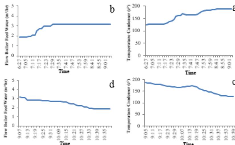
در ناحیه مبرد قبل و بعد از وقوع پدیده طغیان b و کاهش دما a شکل ۶ افزایش دما
