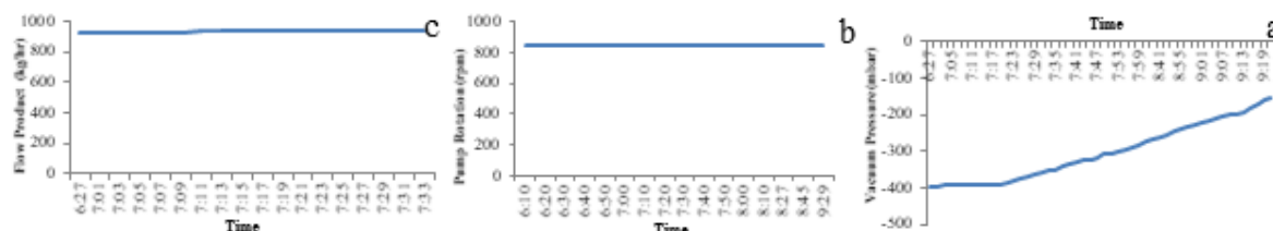
شکل ۷ افت فشار خلأ بالای برج تقطیر a، ثابت بودن تعداد دوران پمپ خلأ b و دبی محصول خالص c هنگام وقوع پدیده طغیان
