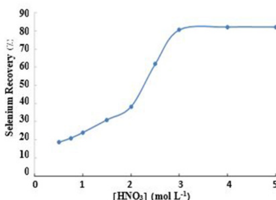
شکل ۲ تأثیر غلظت اسید نیتریک بر بازده فروشویی و بازیابی سلنیم [دما ۷۰ °C، نسبت جامد به مایع (W/V) ۰/۰۲، سرعت هم زدن ۲۰۰ rpm، زمان فروشویی ۴۵ دقیقه] Fig. 2 The effect of Nitric Acid concentration on leaching and recovery of selenium [Temperature 70°C, S/L 0.02 (w/v), stirring speed 200 rpm, leaching time 45min]
